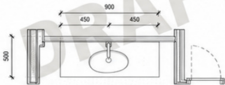
4 PLAN - ENSUITE 2 VANITY 1 : 20
