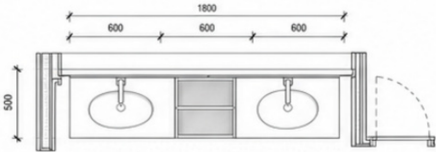
1 PLAN - ENSUITE 1 VANITY 1 : 20
