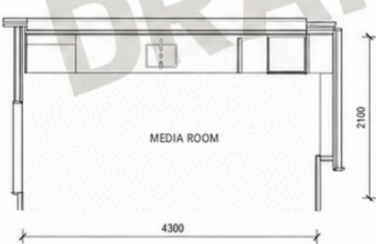
4 PLAN - MEDIA KITCHENETTE 1 : 50
