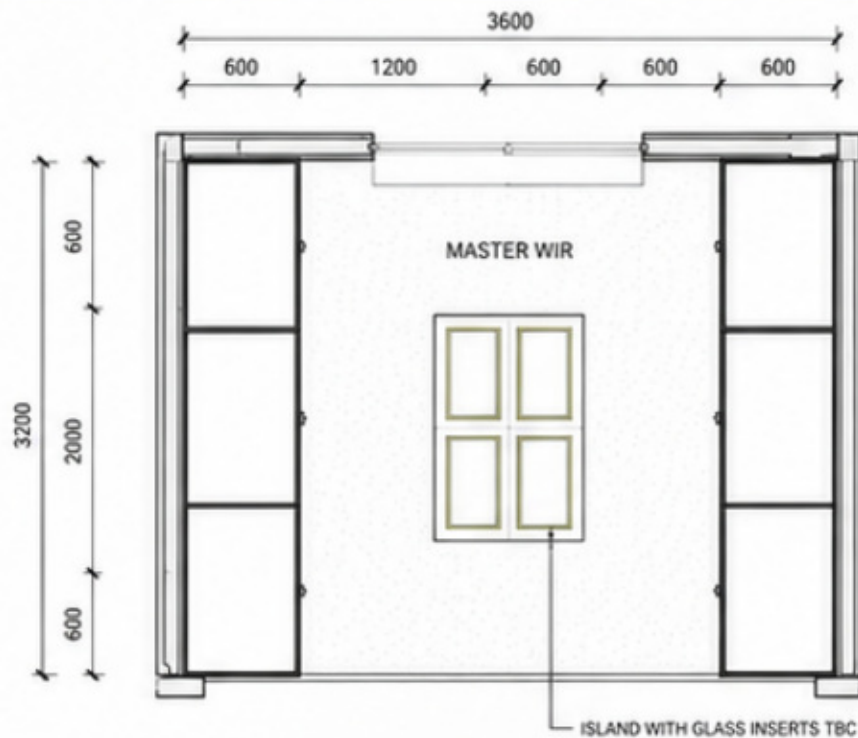
1 PLAN - MASTER WIR 1 : 50
